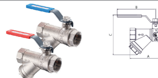
ZAWÓR GW/GW Z FILTREM, DŹWIGNIA
